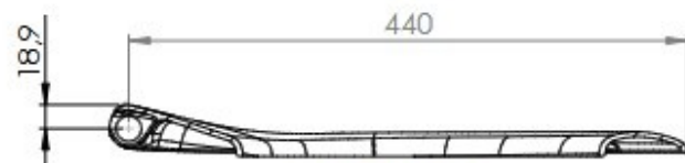
SCHNITT C-C
