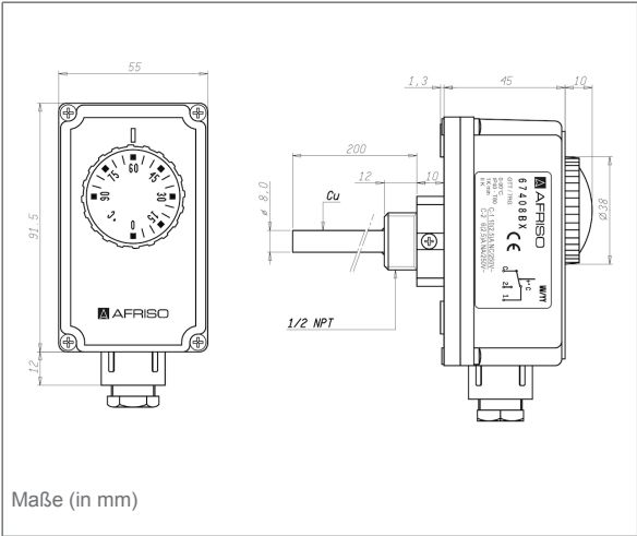
GTT/7RG, Verstellung außenliegend
