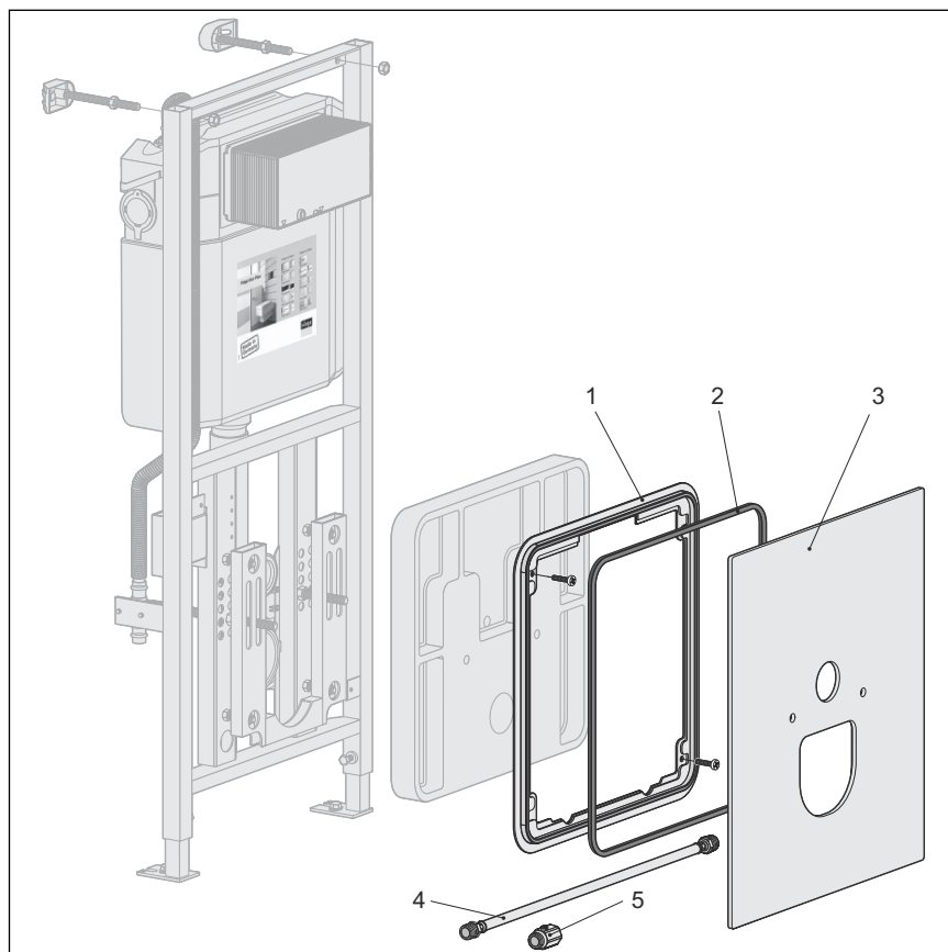
Abb. 1: Bauteile Abdeckplatte Modell 8040.17
