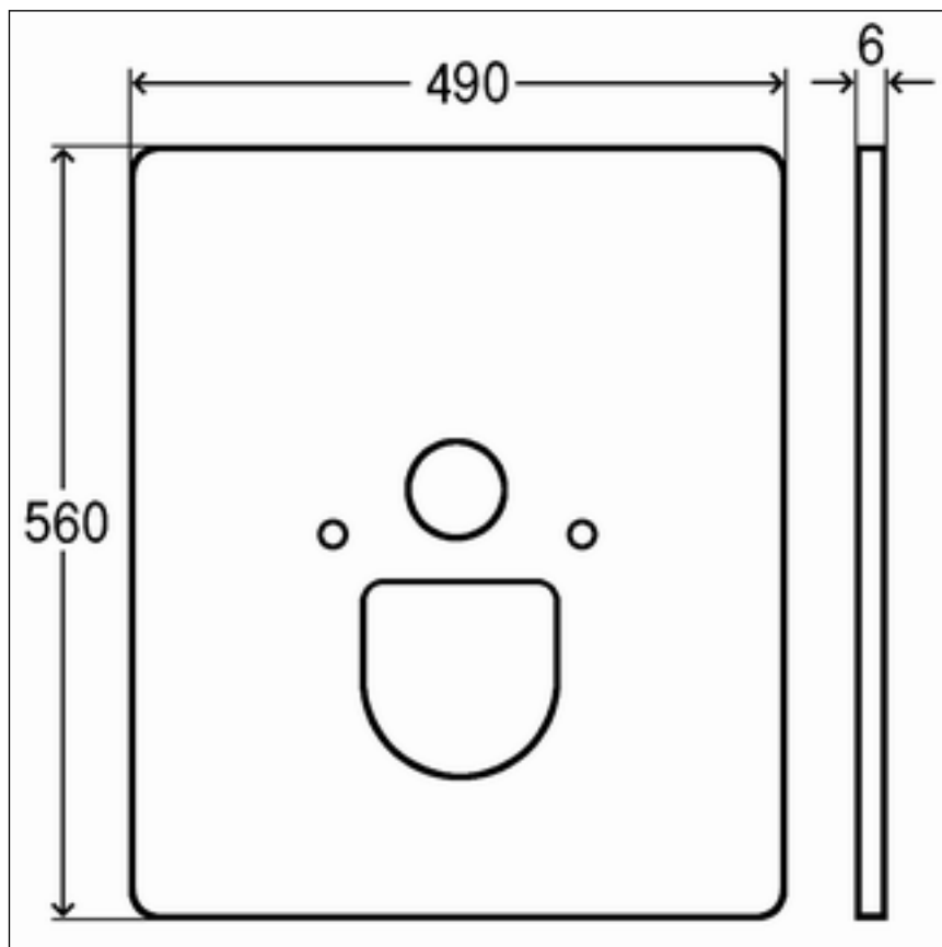
Abb. 2: Abmessungen Abdeckplatte Modell 8040.17
