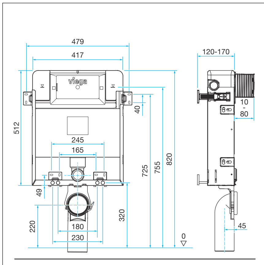
Abb. 1: Maßzeichnung
