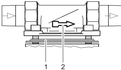
Abb. 5: Einbaudrehflansch
