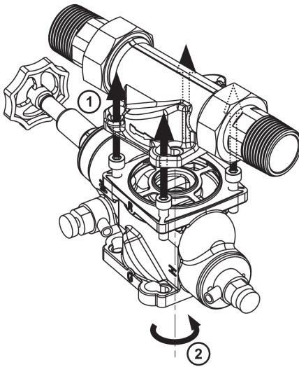
Abb. 8: Schrauben durchführen und einrasten
