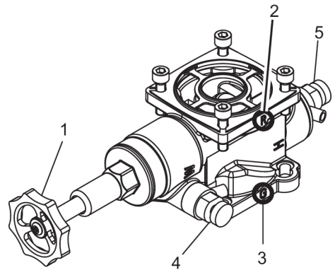
Abb. 7: Umgehungsventil JQX
