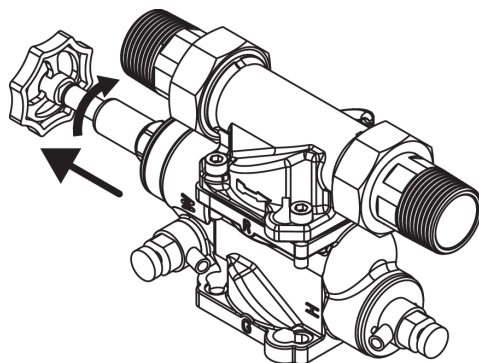
Abb. 17: Normaler Betriebszustand: das Handrad aufdrehen, bzw. bei Montage wie abgebildet nach hinten drehen, bis zum Anschlag.
