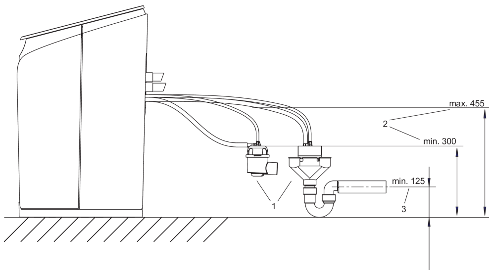
Abb. 14: Korrekte Platzierung des Siphons (Maße in mm)
