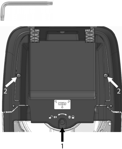
Abb. 10: Abdeckplatte entfernen
