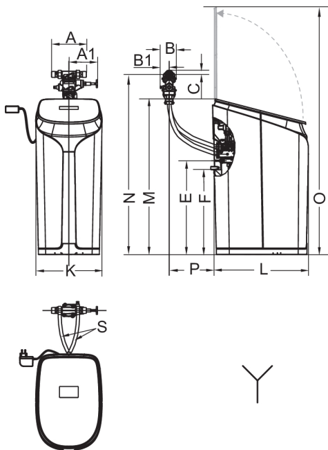
Abb. 21: Einbaumaße i-soft PRO
