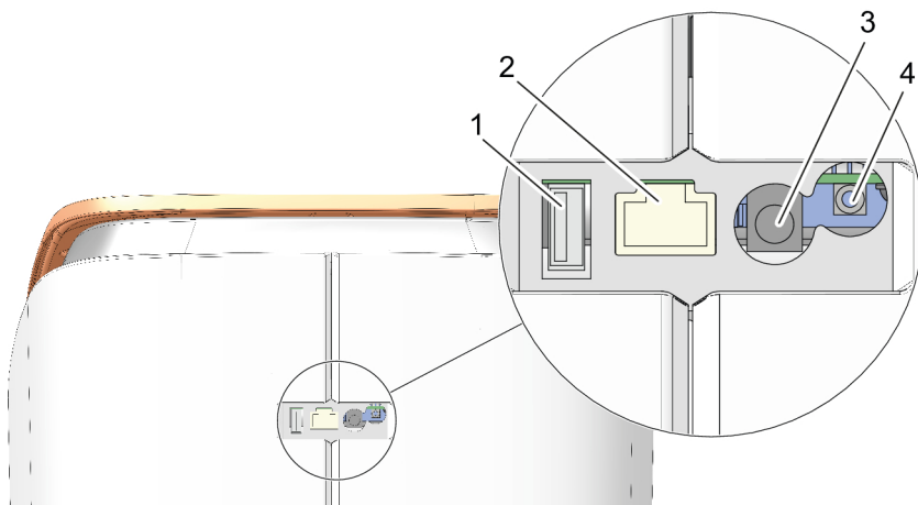
Abb. 3: Anschlussmöglichkeiten auf der Rückseite
