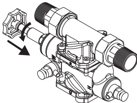
Abb. 16: Auf Umgehung stellen: das Handrad zudrehen, bzw. bei Montage wie abgebildet nach vorne drehen, bis zum Anschlag.
