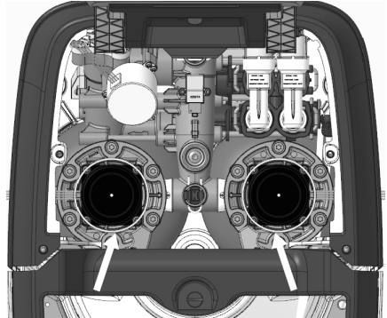
Abb. 12: Transportsicherungen nach oben abziehen
