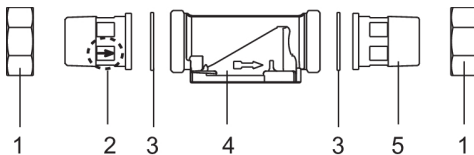
Abb. 6: Einbaudrehflansch, Bestandteile
