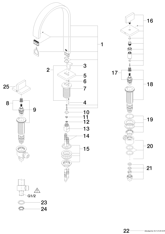
22 — Ablaufgarnitur 8431101.020.0014
