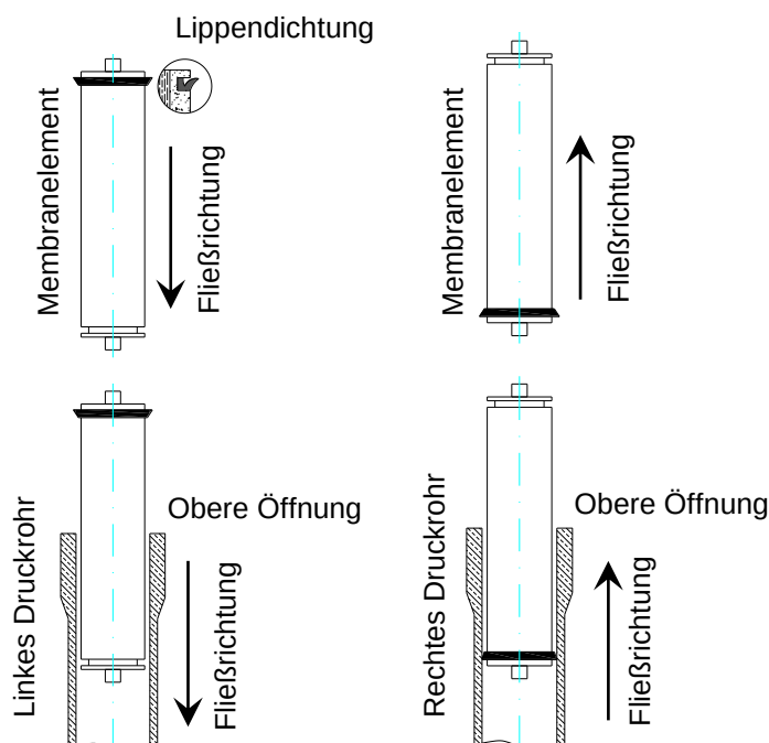
Abb. 12: Membranelemente in Druckrohre einführen (Frontansicht der Anlage)
