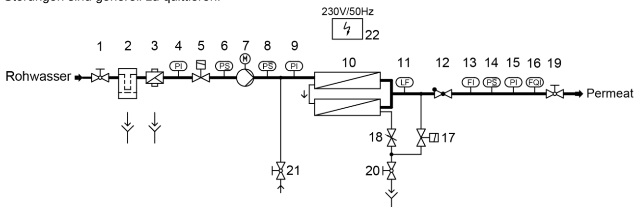
Abb. 1: Funktionsschema
