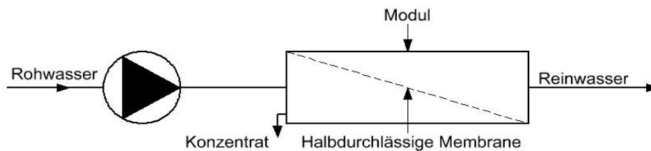
Abb. 2: Prinzip Umkehr-Osmose-Anlage
