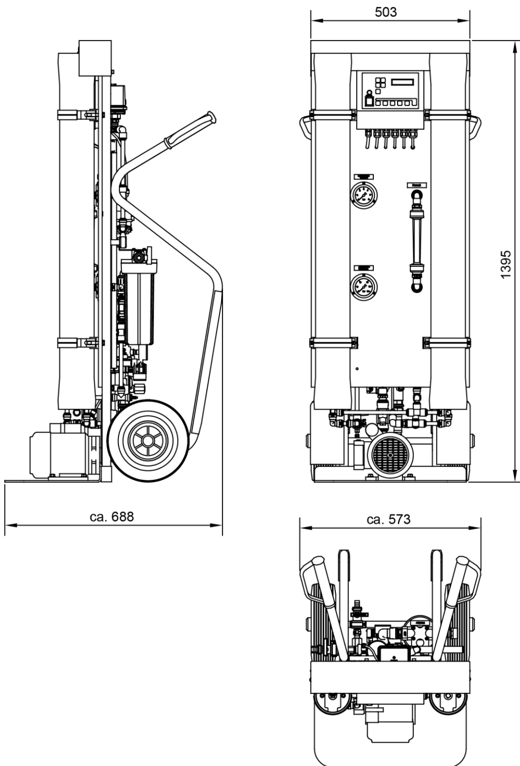
Abb. 4: Abmessungen
