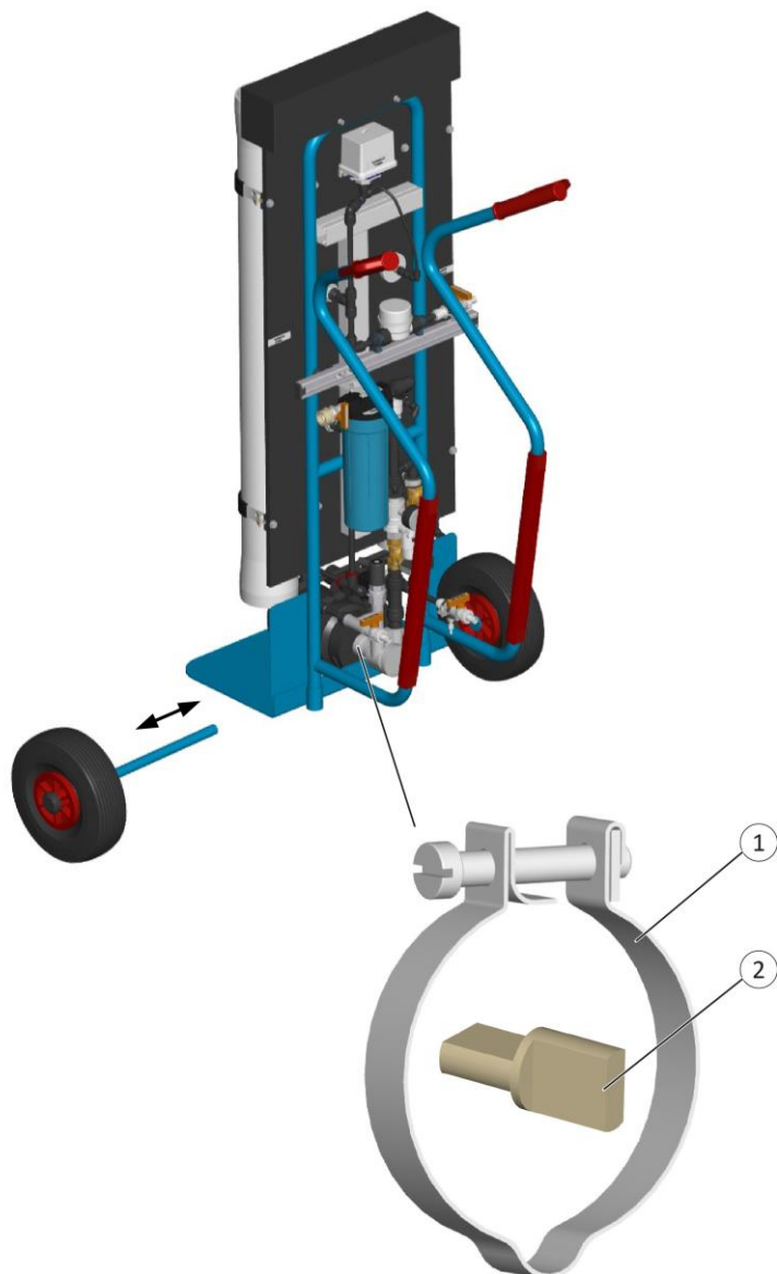
Abb. 12: Detailansicht Kupplungsset
