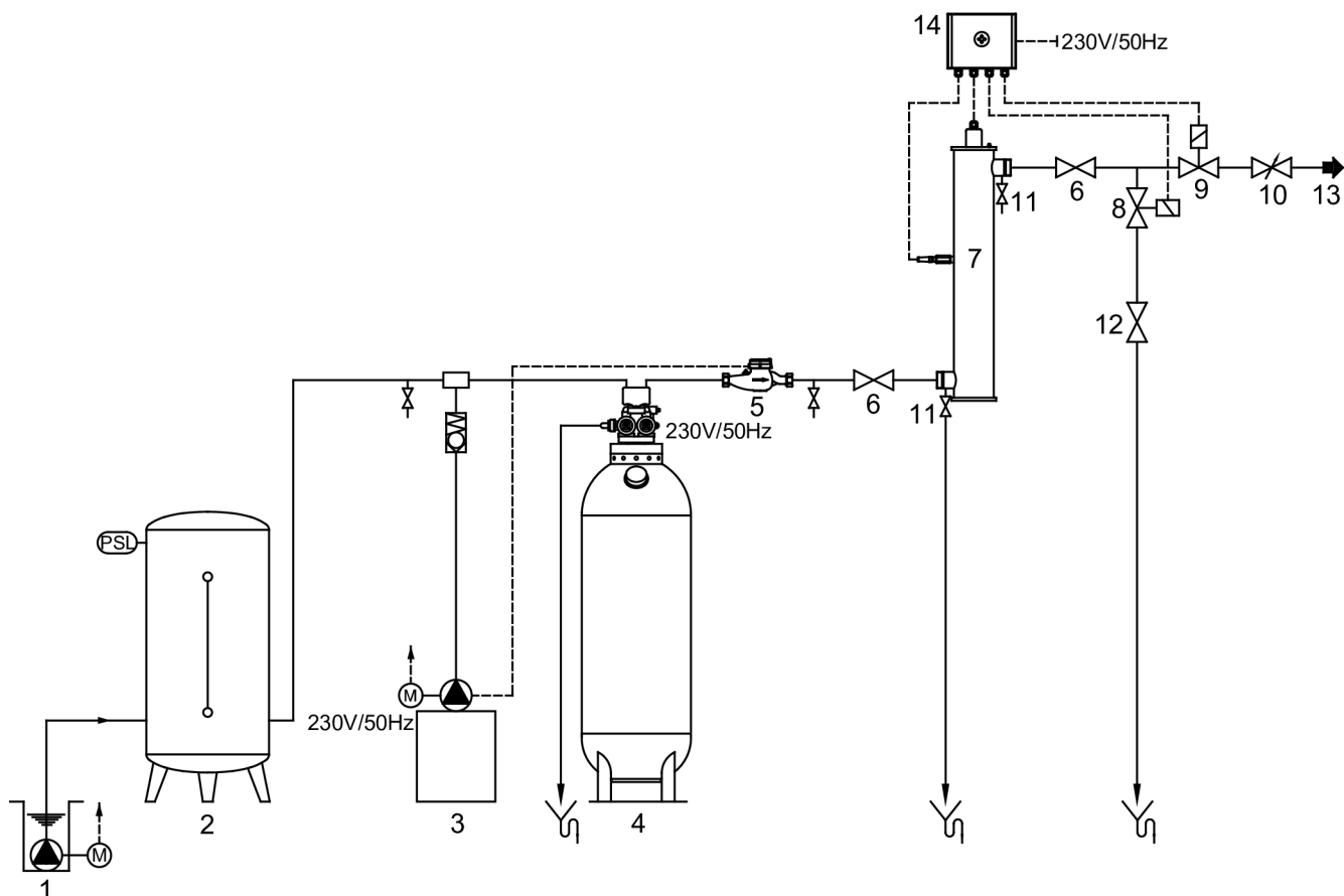
Abb. 6: Installationsbeispiel
