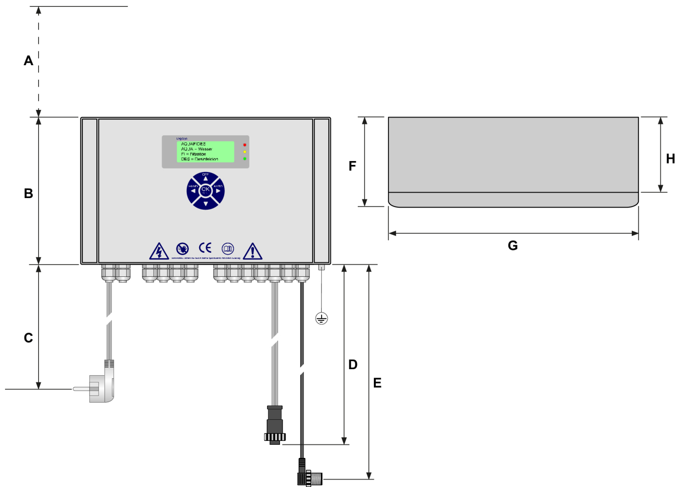
Abb. 3: Abmessungen Steuerung
