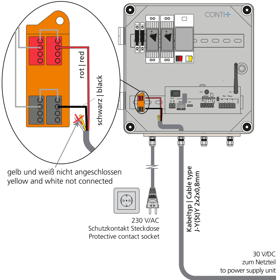
CNX Steuerschrank CNX Control cabinet
