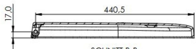
SCHNITT B-B
