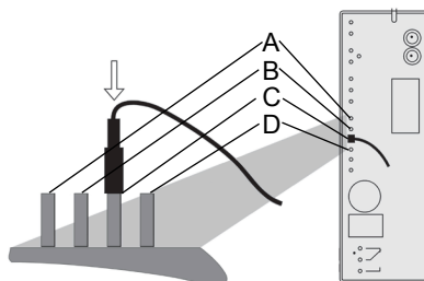
Abb. 3: Zeitsteuerung
