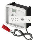
Schaltgerät ACO Multi Control Mono Professional inkl. Staudruckglocke Mit Modbus RTU - Funktionalität zum Anschluss an die Gebäudeleittechnik
