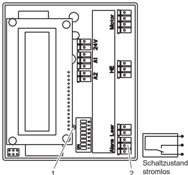
Abb. 23: Elektronische Steuerung
