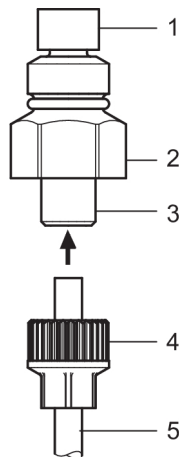
Abb. 15: Impfstück
