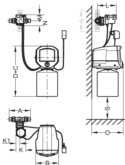
Abb. 20: Einbaumaße i-dos eco 3 / 4 mit externem Wasserzähler
