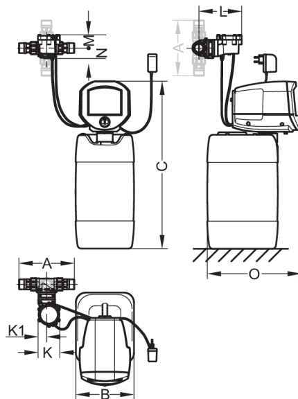
Abb. 21: Einbaumaße i-dos eco 10
