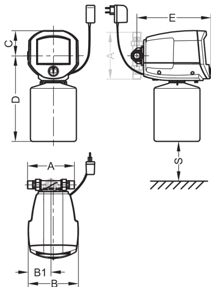
Abb. 19: Einbaumaße i-dos eco 3 / 4 mit integriertem Wasserzähler
