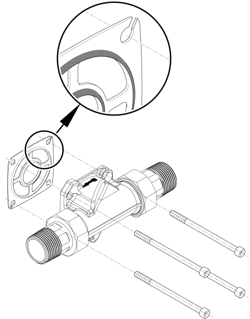
Abb. 5: Profil der Dichtung zum Einbaudrehflansch richten
