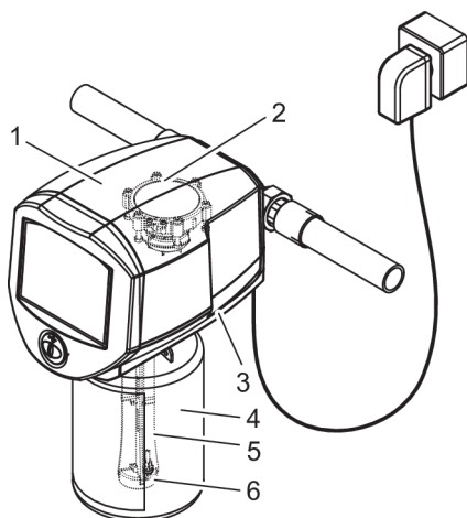
Abb. 6: Einbau i-dos 3 - 4 mit integriertem Wasserzähler
