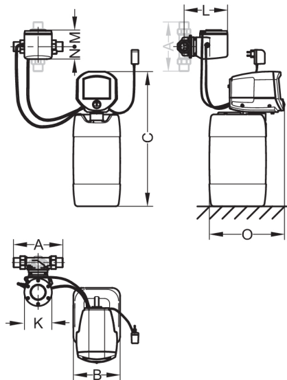
Abb. 22: Einbaumaße i-dos eco 25 / 60
