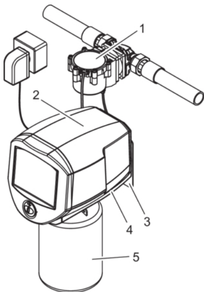
Abb. 9: Einbau i-dos eco 3-4 mit getrenntem Wasserzähler
