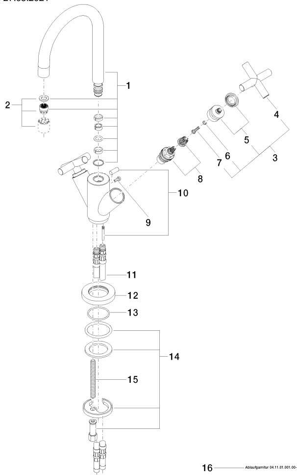
16 — Ablaufgarnitur 04.11.01.001.00-ff
