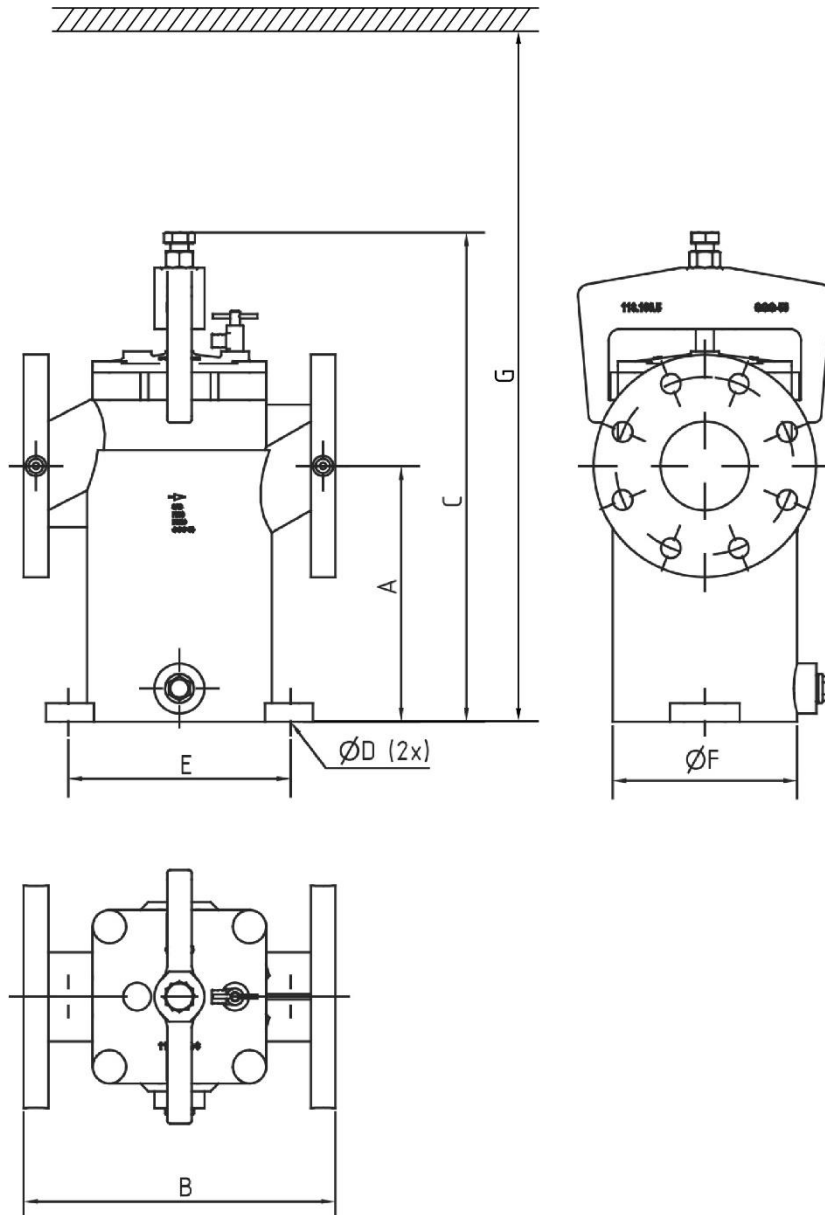
Abb. 3: Maßzeichnung
