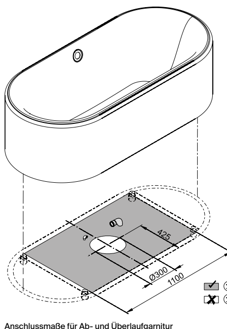
Anschlussmaße für Ab- und Überlaufgarnitur
