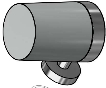
Adapter \varnothing 41 \times 8 PB20-PRO
