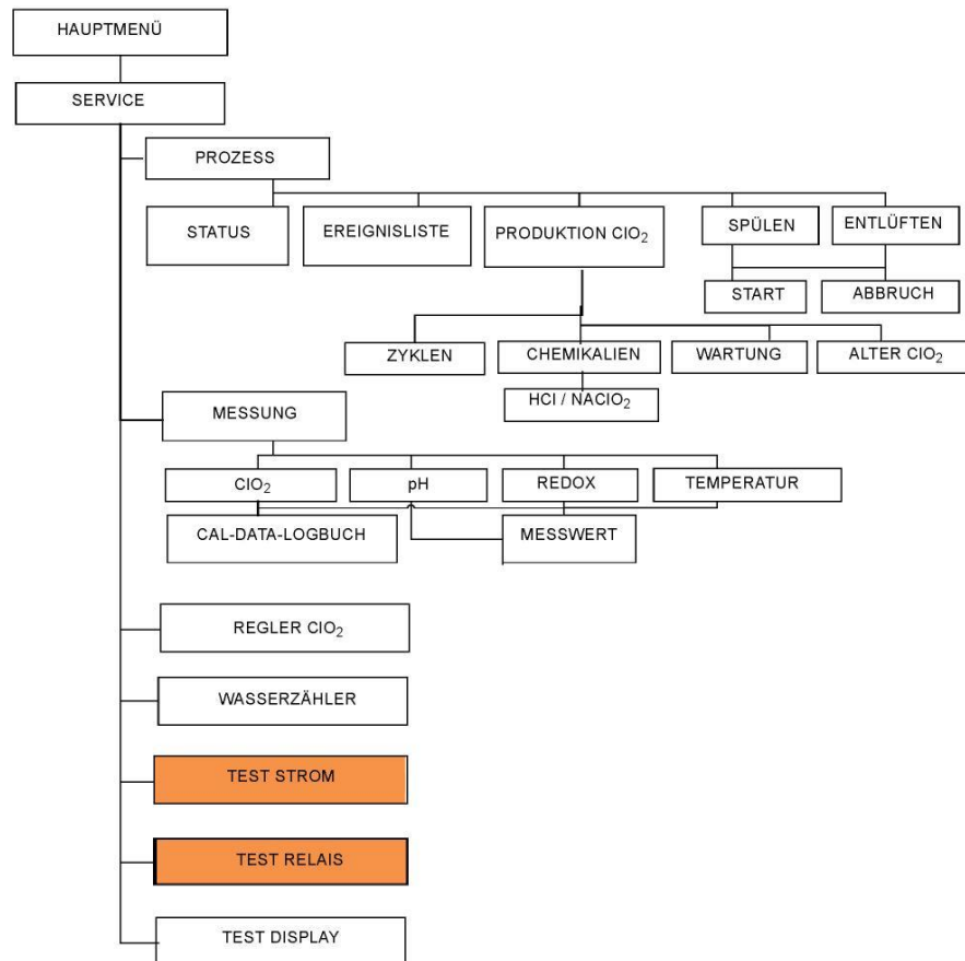
Abb. 13: Menüstruktur Service-Menü
