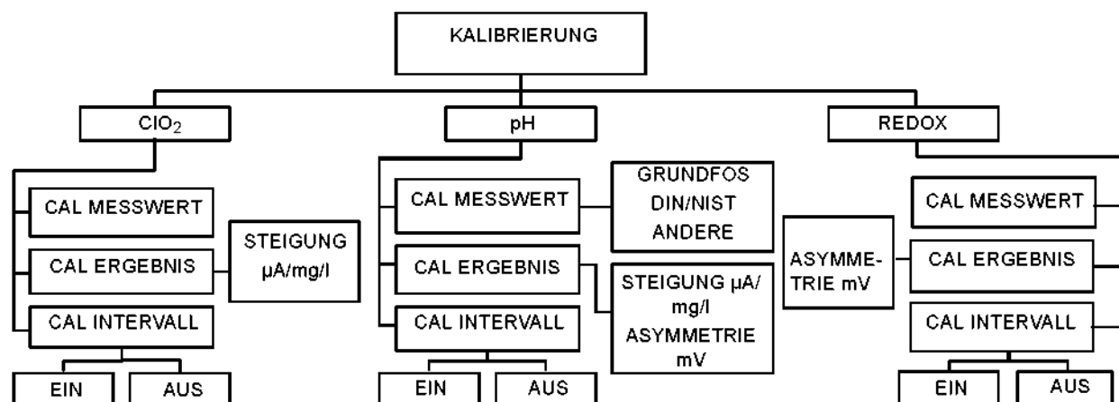
Abb. 15: Menüstruktur Kalibrieren
