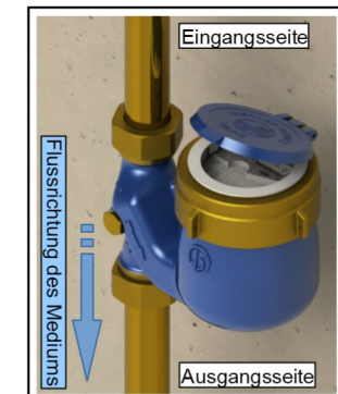
Einbau Fallrohr
