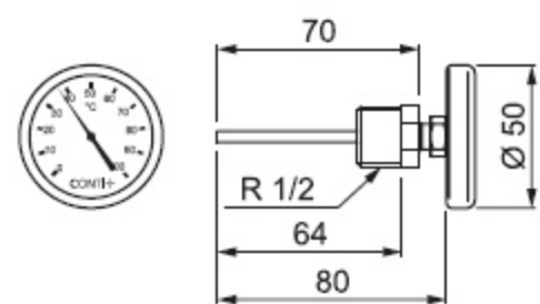
Thermometer mit beiliegendem Reduzierstück 1/2" x 1/4"
