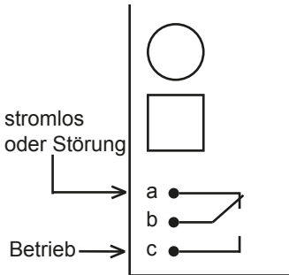
Abb. 5: Belegung Relaiskontakte
