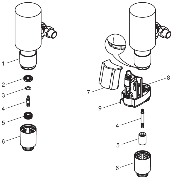
Abb. 1: Montage des Automatik-Nachrücksatzes
